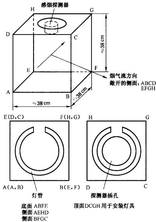
图 C.1 闪光装置图
