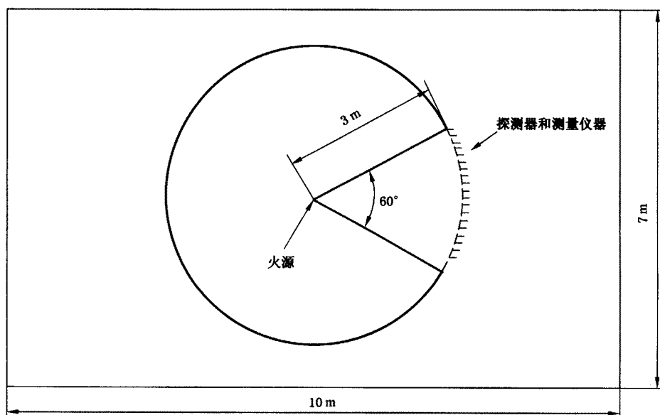
图 F.1 试验布置图
