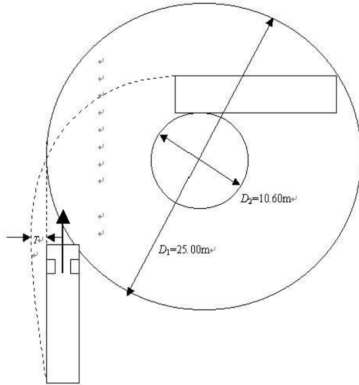
图 A.1 车辆通道圆与外摆值示意图(汽车) GB 1589-2004
